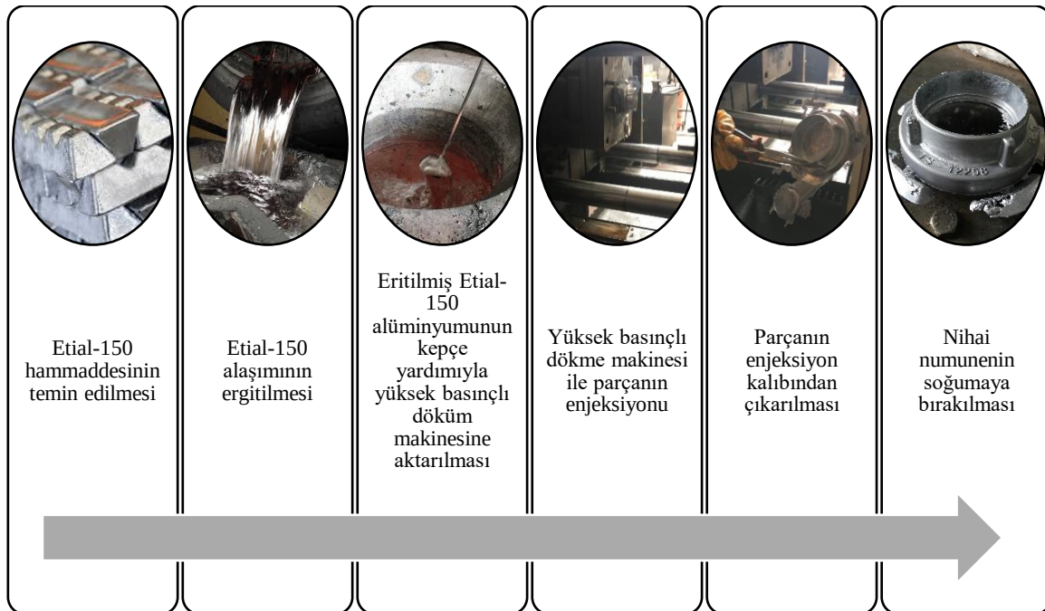
Şekil 1. Üretim yönteminin akış şeması
