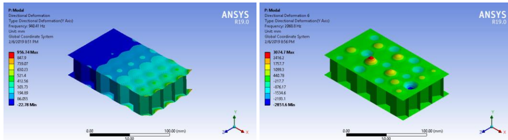
Şekil 6. C=20 H=30 4x Model Yerçekimi Öngerilmeli Bal Peteği Kompozit Malzemenin Doğal Frekans Analizi Sonucunda Y Yönünde Ana Mod Salınım Görseli (Solda), Lokal Mod Salınım Görseli (Sagda)
