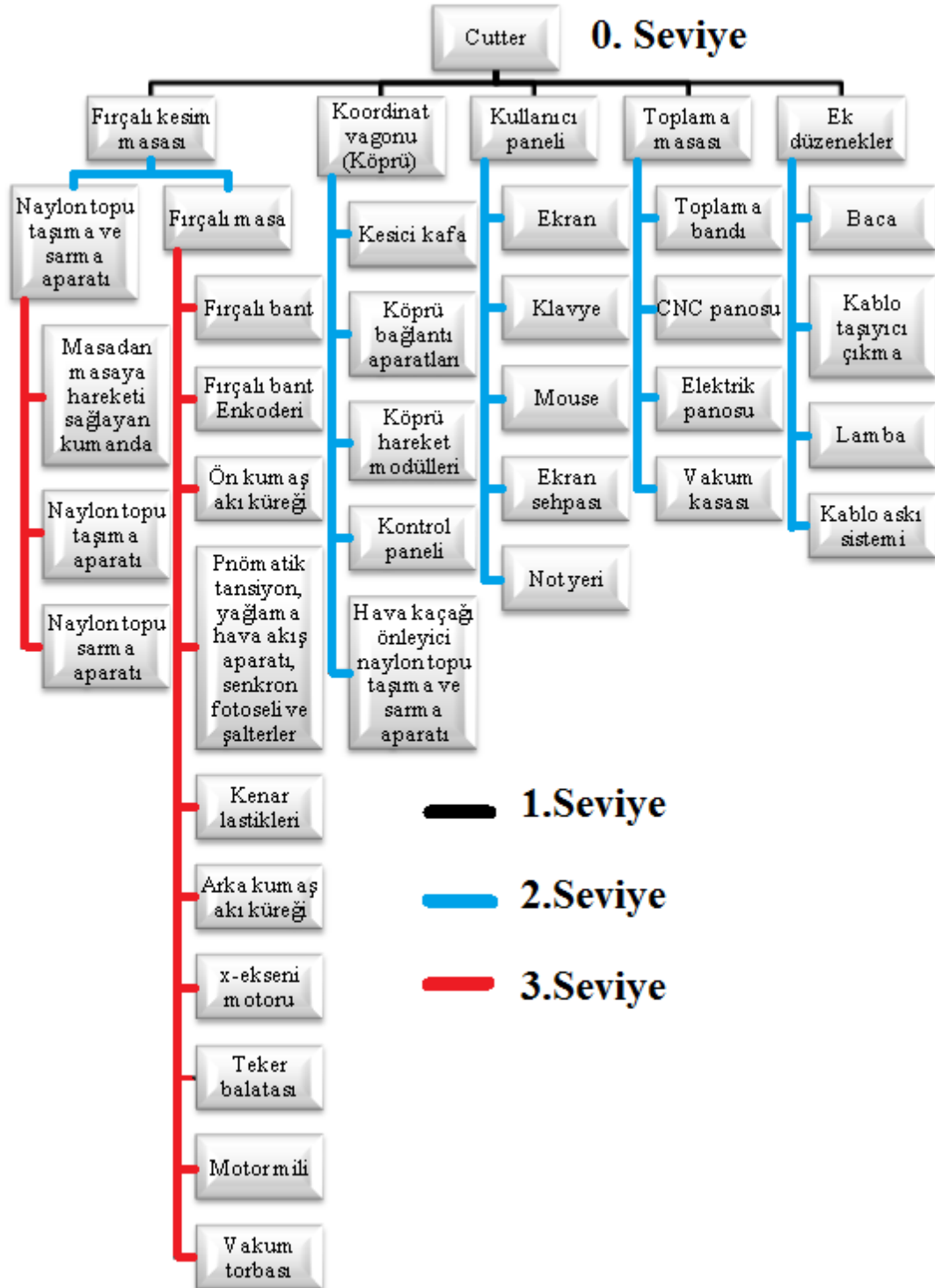
Şekil 4. Assyst Bullmer Cutter Ürün Ağacı (Çetin, M.S., 2011)
