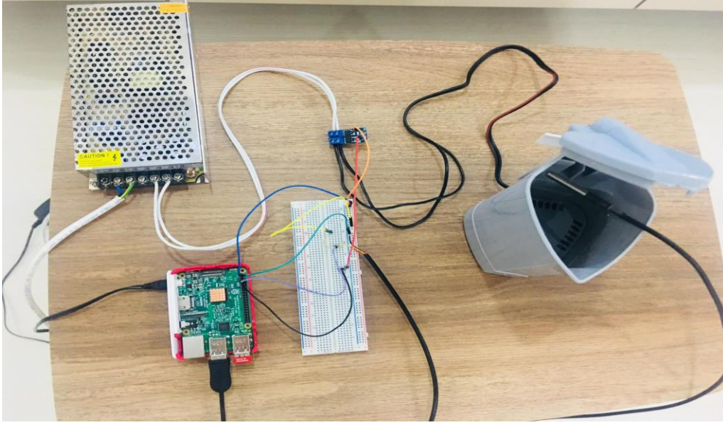
Şekil 9. Sıcaklık kontrol sistemin genel görünüşü
