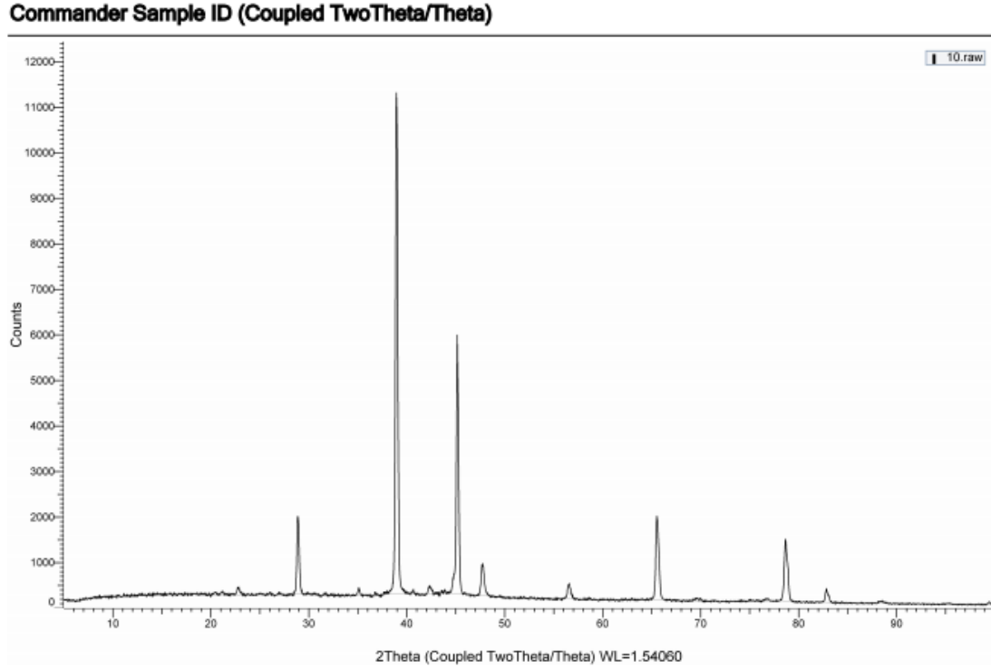
Şekil 3. ETIAL 150 alaşımlarının XRD analizi
