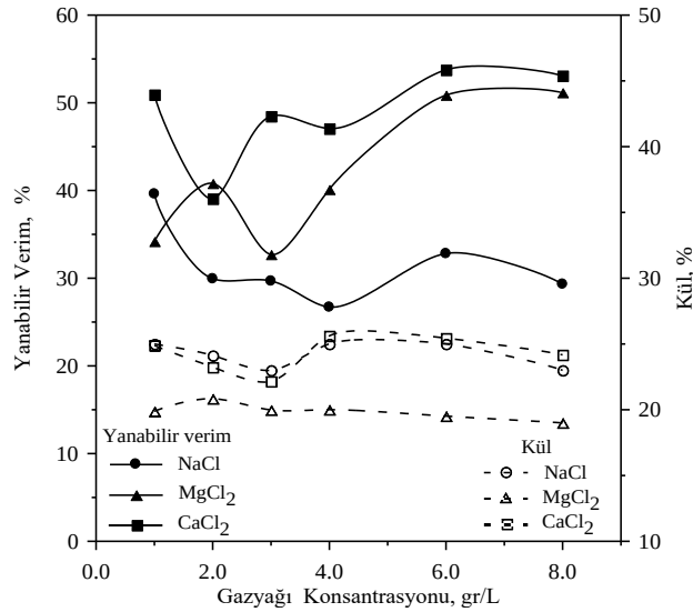
Şekil 6. 10 -1 M NaCl, MgCl 2 ve CaCl 2 Konsantrasyonunda Gazyağı Derişiminin Linyit Flotasyonuna Etkisi.
