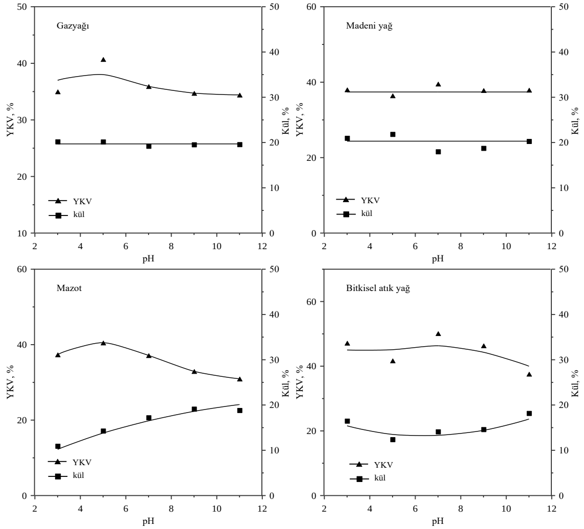
 ekil 2. K m r n farklı yađlarla aglomerasyonuna pH'ın etkisi
