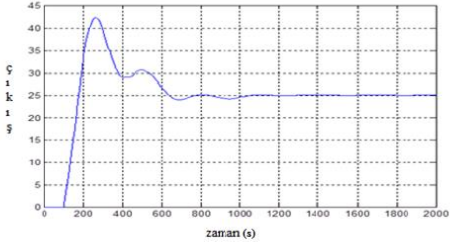
Şekil 6. Sıcaklık kontrol sisteminin basamak cevabı
