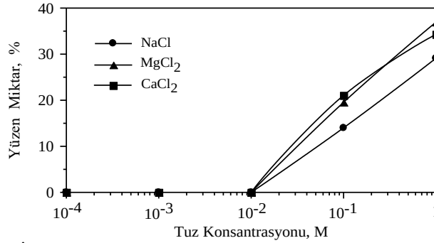
Şekil 2. Farklı İnorganik Tuzların Konsantrasyonuna Bağlı Olarak Linyitin Flotasyonu.
